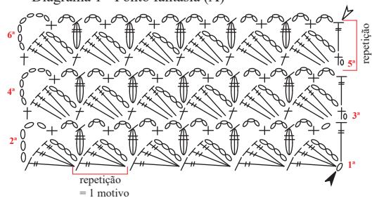
Diagrama 1 - Ponto fantasia (A)
