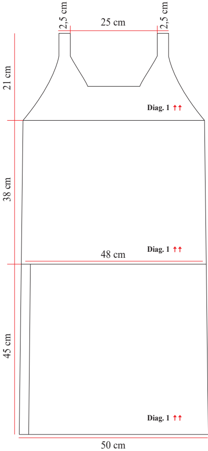
Esquema de medidas Frente = Costas
