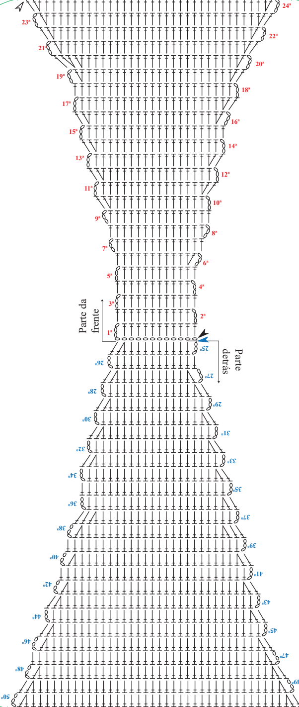
Diagrama 1 - Tanga - (1ª etapa)
